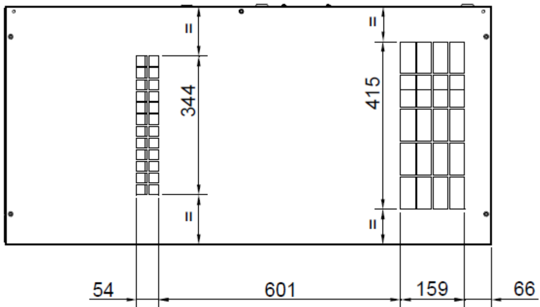
Figura 3 – Vista superior do compressor de ar.
