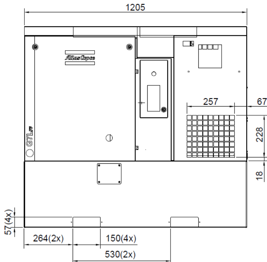
Figura 1 – Vista frontal do compressor de ar.
