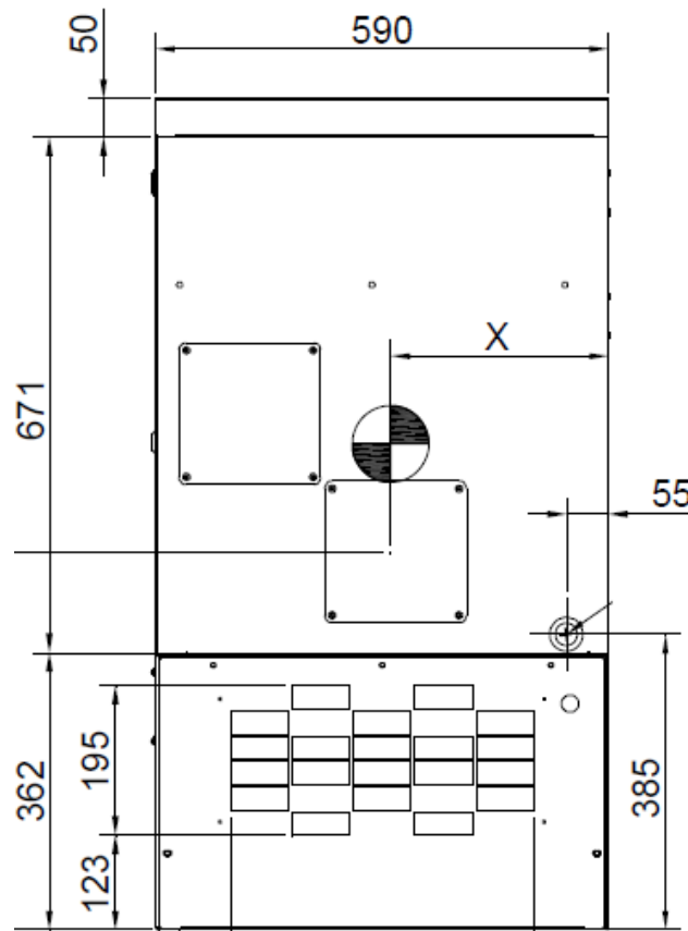
Figura 2 – Vista lateral do compressor de ar.
