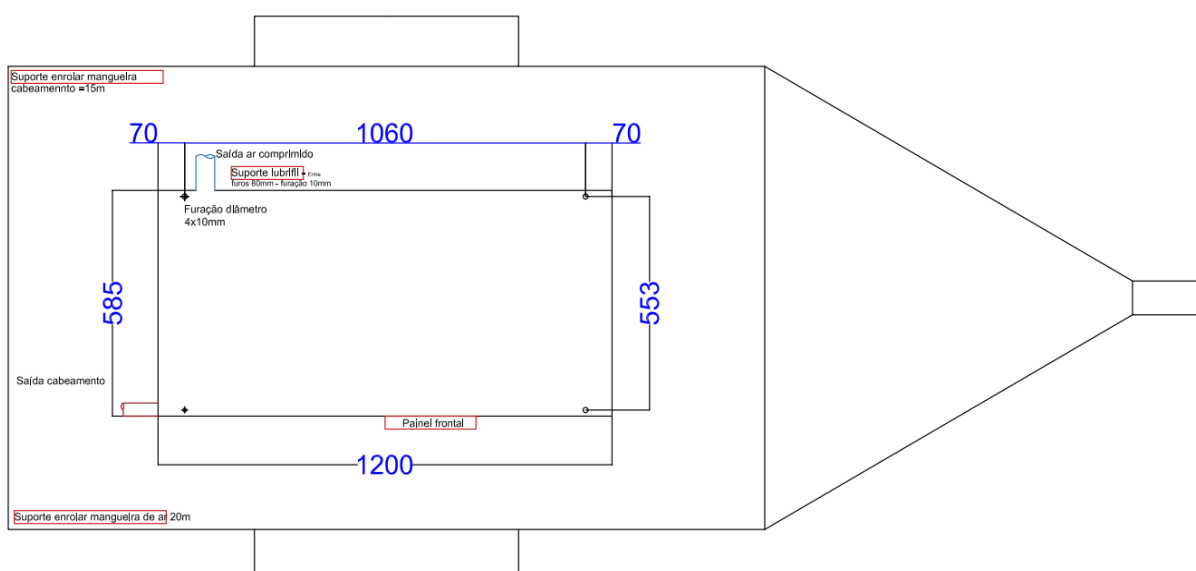
Figura 4 – Vista superior do compressor de ar.
